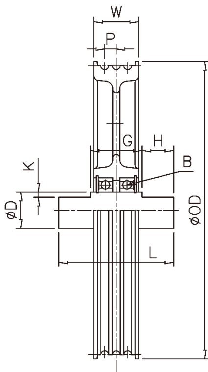
導向輪
