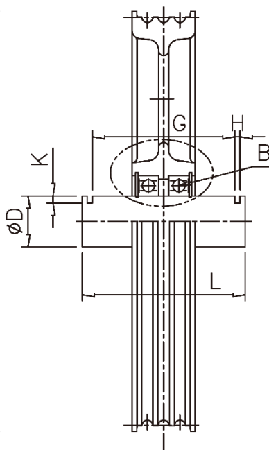
懸吊輪
